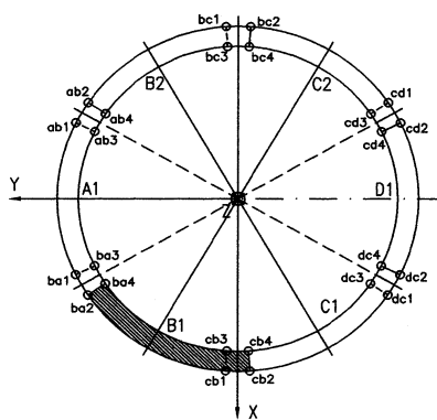
Frontansicht Tübbingring
