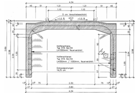
Querschnitt
