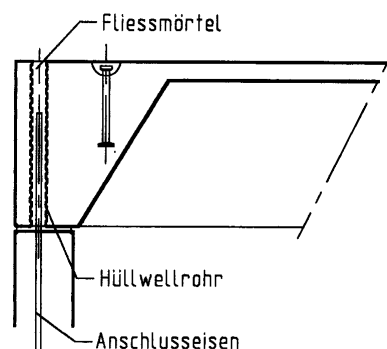
Anschlussdetail Rippenplatte-Wand mit Endblockausbildung
